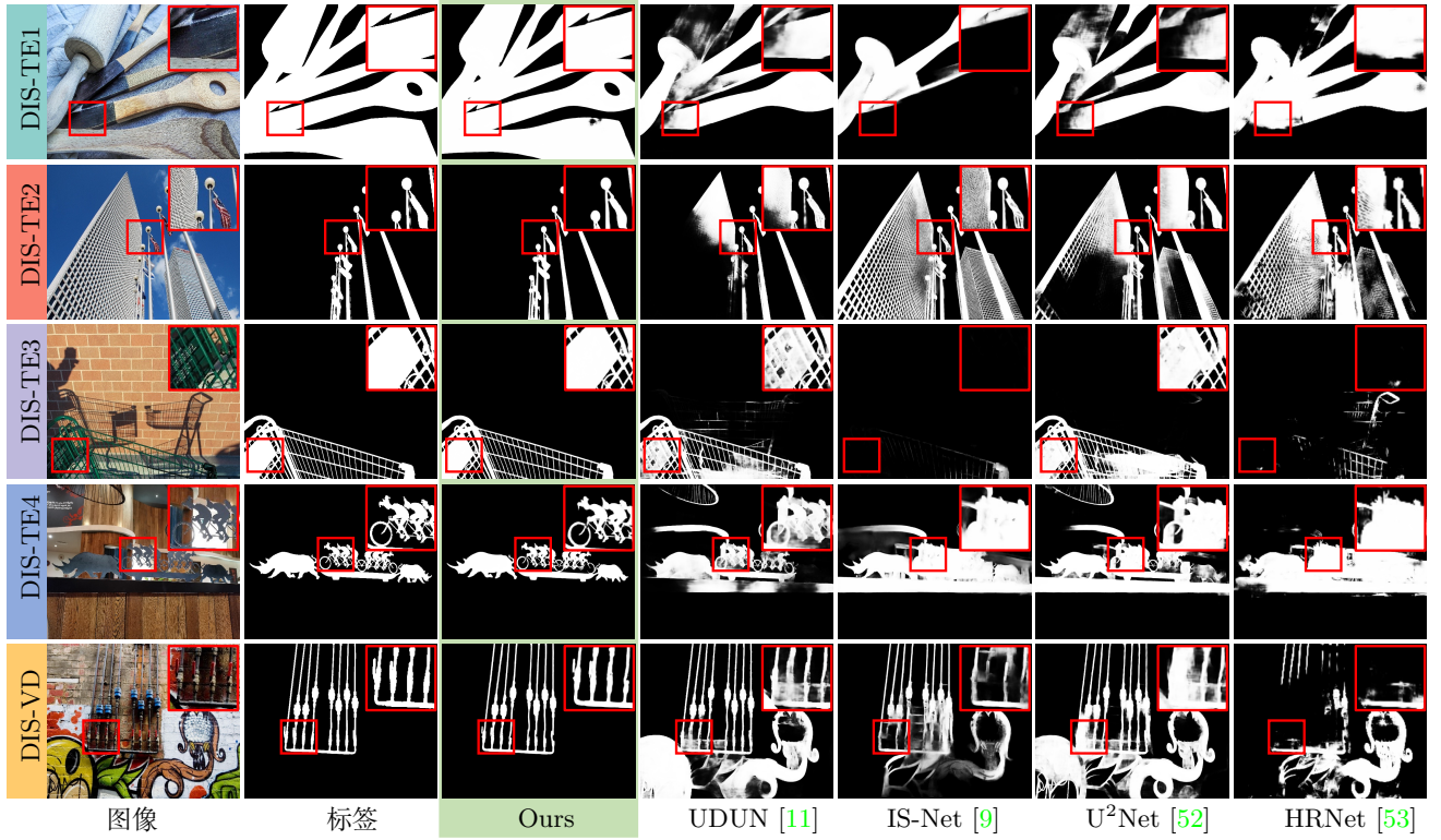
图 5 所提出的 BiRefNet 在 DIS5K 数据集上与先前方法的定性比较。先前方法的结果来源于文献 [11]，其中所有模型均使用 1024×1024 大小的图像进行训练。放大以获得更好的视图。
