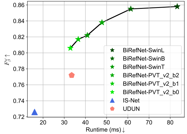
图 8 BiRefNet 与现有 DIS 方法在效率、规模、复杂性和性能方面的比较。
