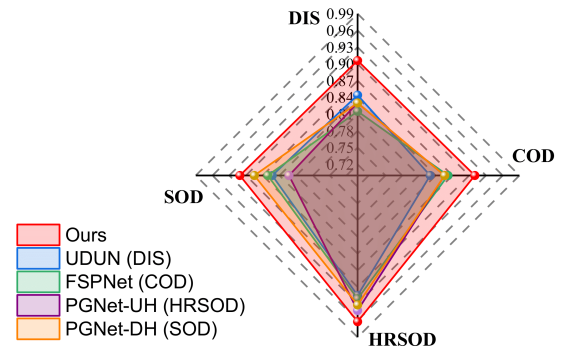
图 7 提出的 BiRefNet 与最佳任务特定模型的定量比较。这里使用 S-measure [12] 进行比较。UDUN [11]、FSPNet [23]、PGNet-UH [14] 和 PGNet-DH [14] 分别是目前在 DIS、COD、HRSOD 和 SOD 任务上的最佳模型。
