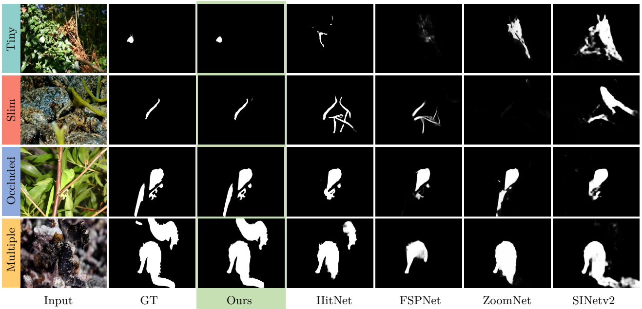
图 6 在 COD10K 基准测试上，提出的 BiRefNet 与其他竞争方法的视觉比较。这里提供了具有不同挑战性的样本，以展示 BiRefNet 在不同视角上的优越性。
