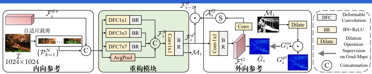
图 4 提出的双边参考块的流程。原始尺度的源图像与解码器特征结合作为内部参考，输入重建块中，采用具有层次感受野的可变形卷积。聚合的特征然后用于预测外部参考中的梯度图。梯度感知特征然后被转换为注意力图，作用于原始特征。
