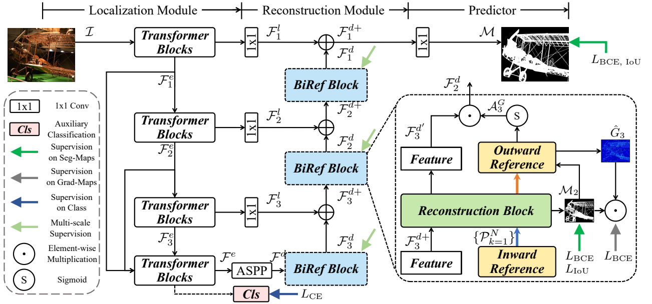
图 3 所提出的双边参考网络 (BiRefNet) 的流程图。BiRefNet 主要由定位模块 (LM) 和具有双边参考 (BiRef) 块的重建模块 (RM) 组成。详细信息请参见 Sec. 3.1。
