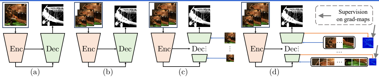
图 2 我们提出的 BiRefNet 与其他现有高分辨率分割任务方法的比较。(a) 常见框架 [1]; (b) 图像金字塔作为输入 [2,3]; (c) 缩放后的图像作为内部参考 [4,5]; (d) BiRefNet: 原始尺度图像的块作为内部参考, 梯度先验作为外部参考。Enc = 编码器, Dec = 解码器。
